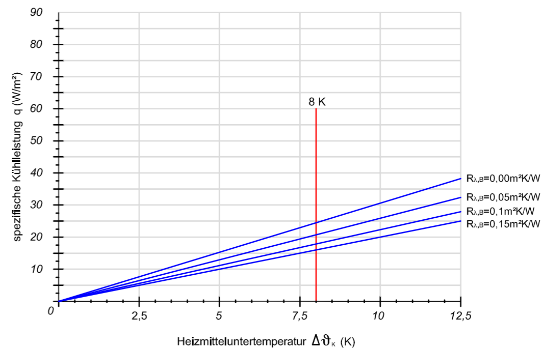
Verlegeabstand VA 250
