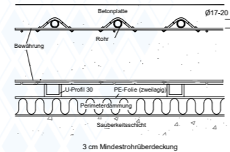
3 cm Mindestrohrüberdeckung
