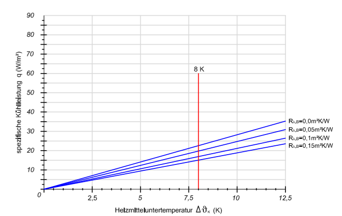
Verlegeabstand VA 300
