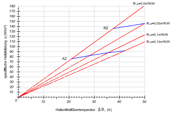
Verlegeabstand VA 300
