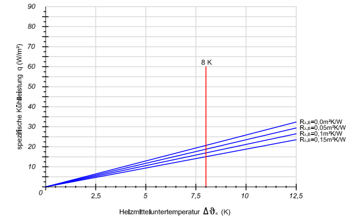
Verlegeabstand VA 250
