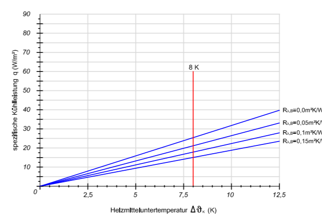
Verlegeabstand VA 250
