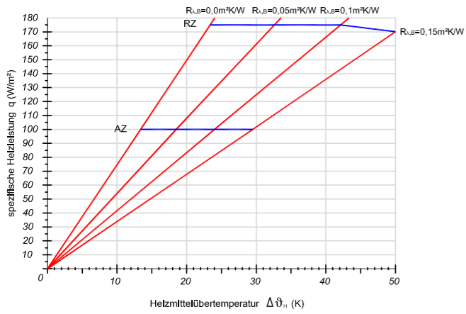
Verlegeabstand VA 50*
