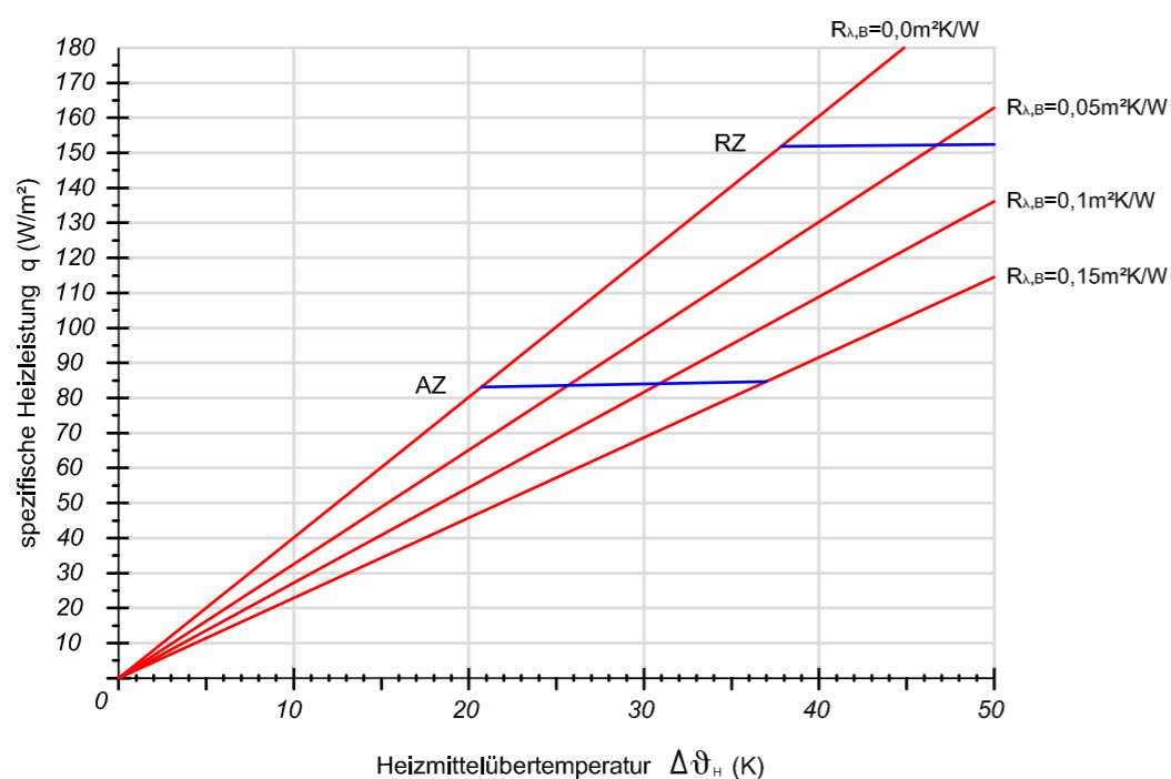
Verlegeabstand VA 250
