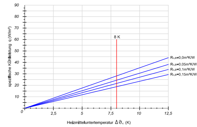
Verlegeabstand VA 100
