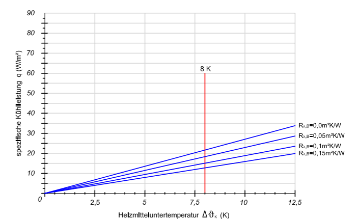
Verlegeabstand VA 300
