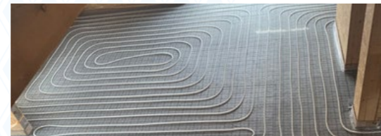
Rohr mit Klettbefestigung
