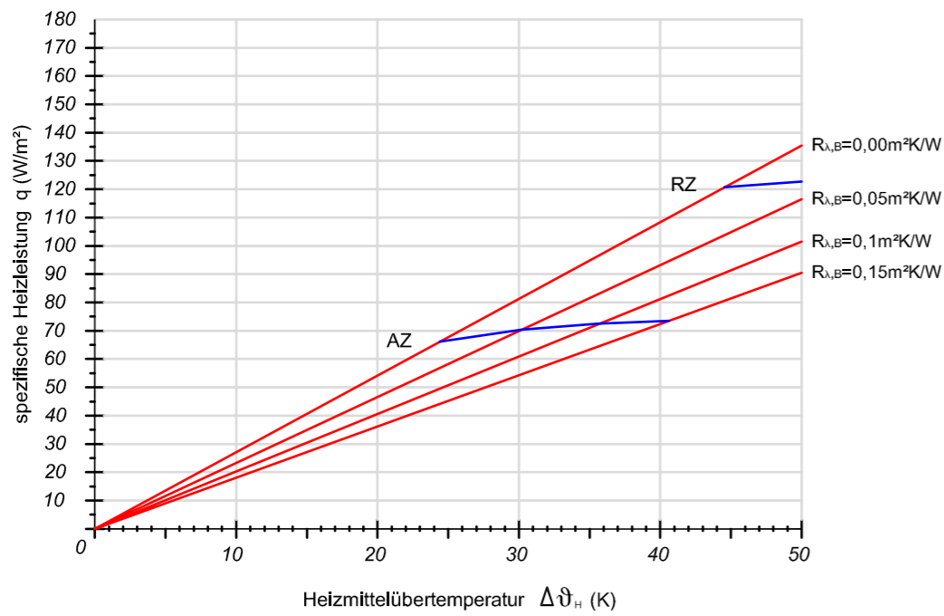
Verlegeabstand VA 250
