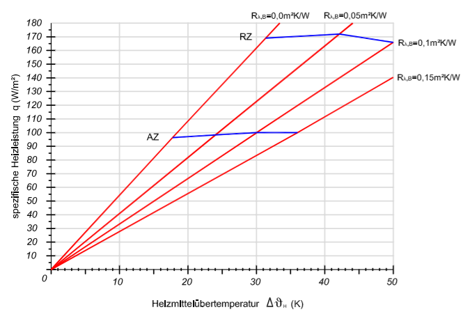
Verlegeabstand VA 150
