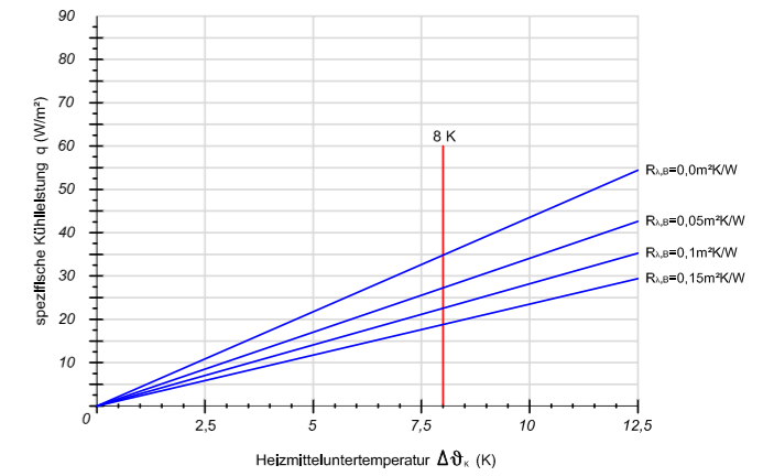
Verlegeabstand VA 100
