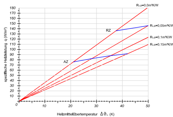
Verlegeabstand VA 300
