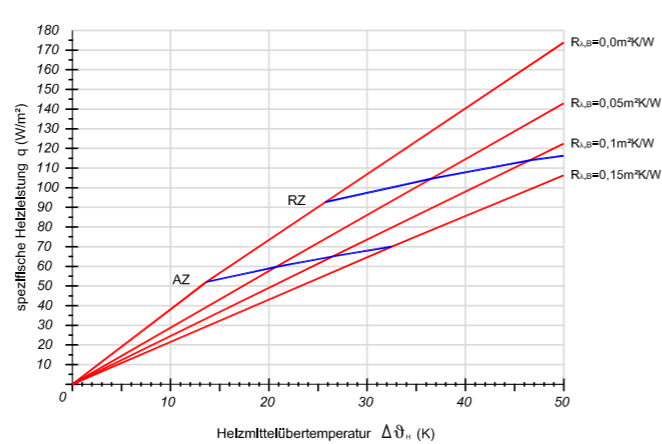
Verlegeabstand VA 350
