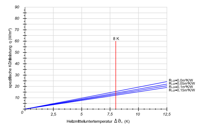
Verlegeabstand VA 350
