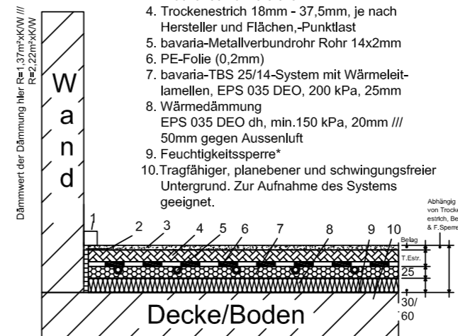
* Bauwerksabdichtung nach DIN 18195 nur gegen Erdreich // ** Höherer Dämmwert empfehlenswert // *** Bei Grundwasserspiegel < 5m höherer Dämmwert empfehlenswert Hinweis: Systemplatte keine Trittschallplatte, Gesamtaufbau z.B. mit Trockenestrich etc. erzeugt Trittschallverbesserung (Massivuntergrund). Holzunterkonstruktion immer situationbedingt.
