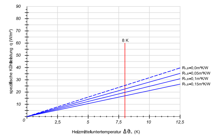
Verlegeabstand VA 250, Pro12
