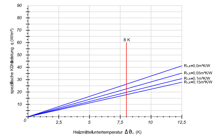
Verlegeabstand VA 150
