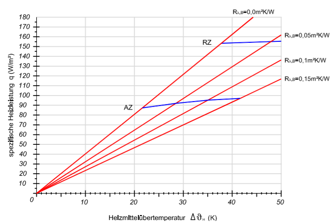
Verlegeabstand VA 250
