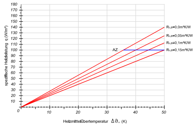
Verlegeabstand VA 250
