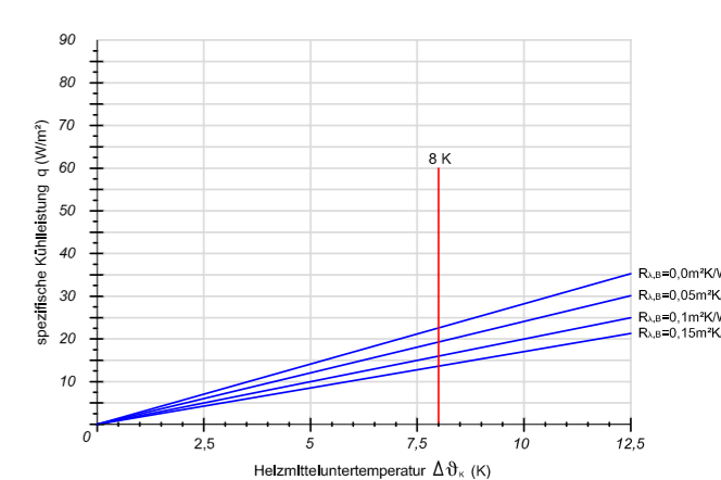
Verlegeabstand VA 300
