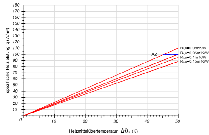
Verlegeabstand VA 350
