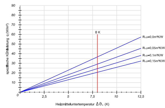
Verlegeabstand VA 100
