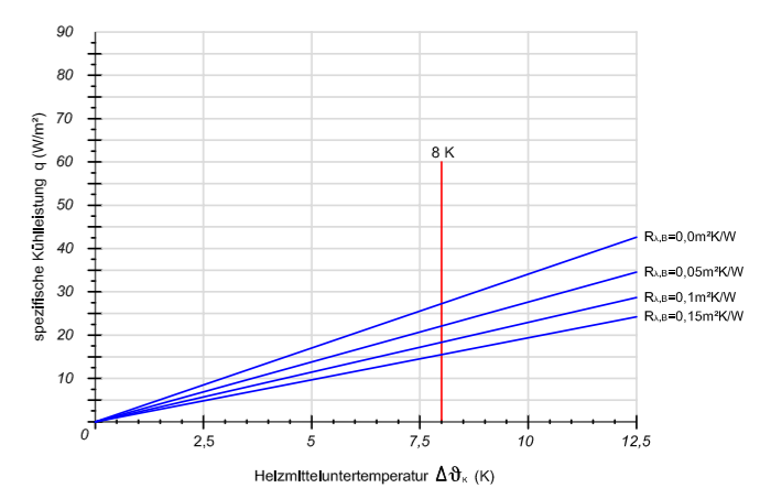
Verlegeabstand VA 200
