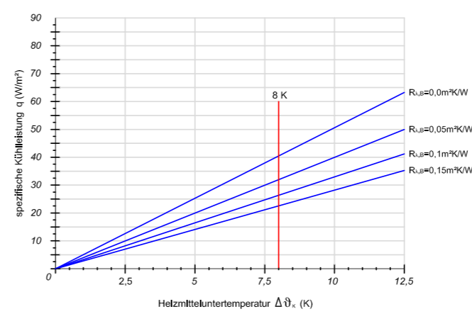
Verlegeabstand VA 50
