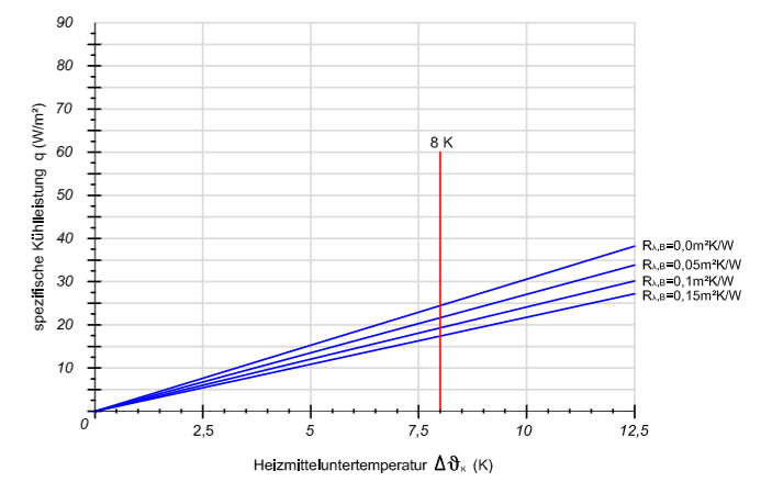
Verlegeabstand VA 150
