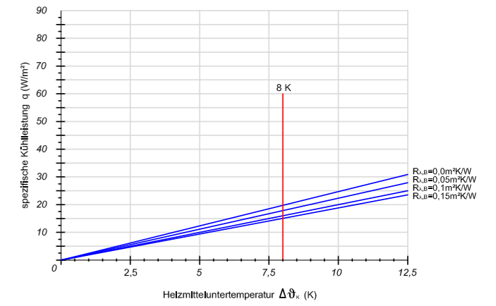
Verlegeabstand VA 250
