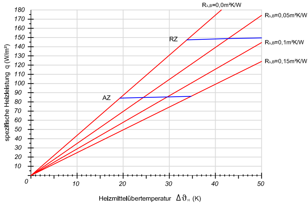
Verlegeabstand VA 125
