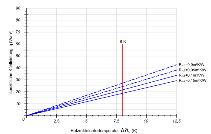
Verlegeabstand VA 250, Expert15
