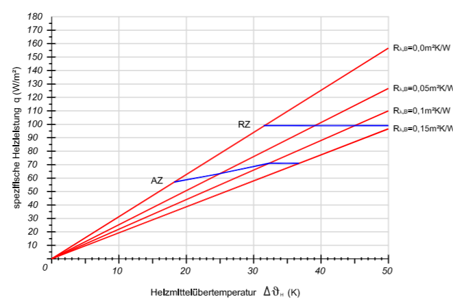
Verlegeabstand VA 350
