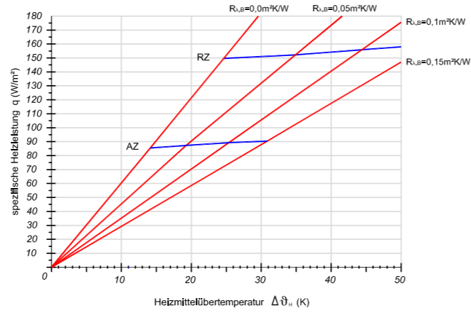
Verlegeabstand VA 150
