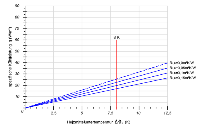
Verlegeabstand VA 250, Pro12
