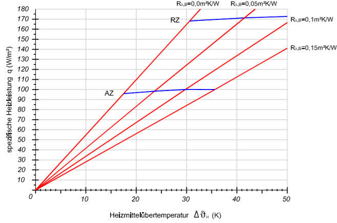
Verlegeabstand VA 150
