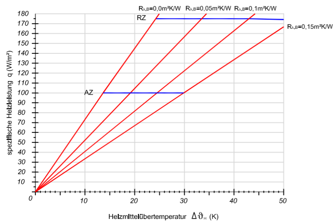
Verlegeabstand VA 50
