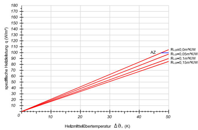
Verlegeabstand VA 350
