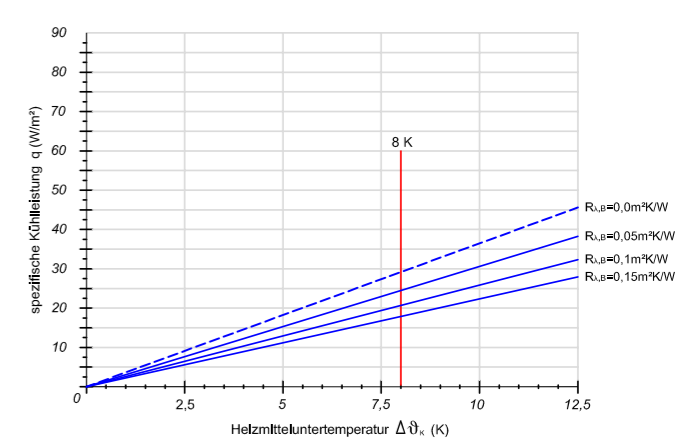
Verlegeabstand VA 250, Strongboard
