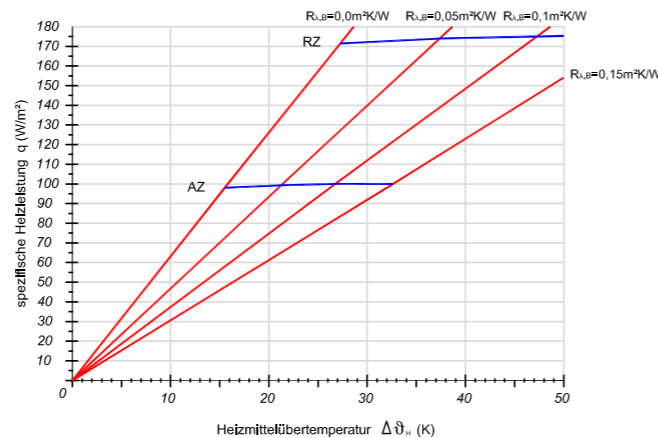
Verlegeabstand VA 100
