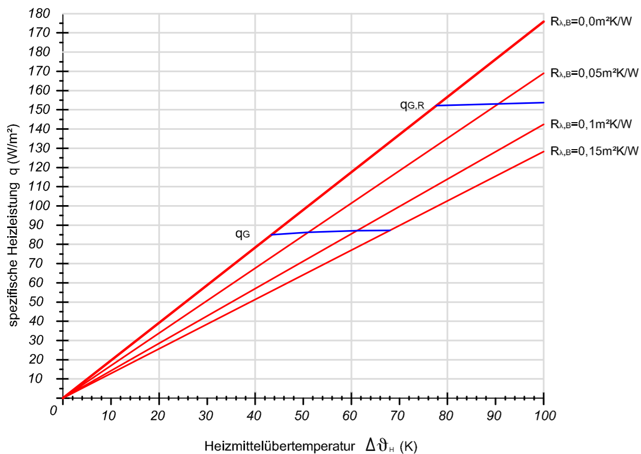
Verlegeabstand VA 125
