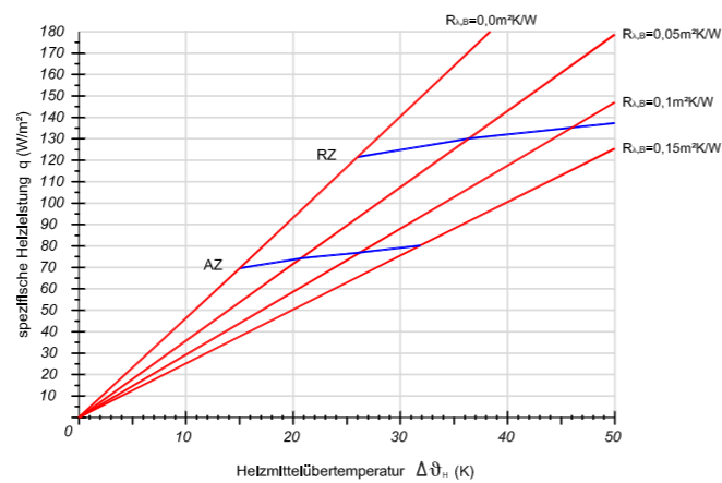
Verlegeabstand VA 250
