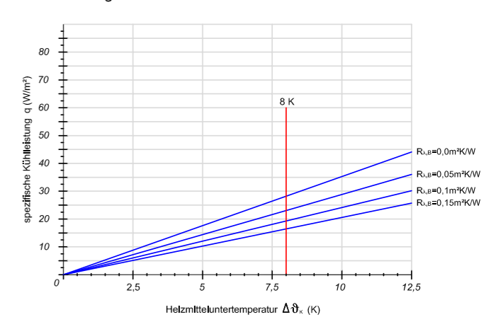
Verlegeabstand VA 200
