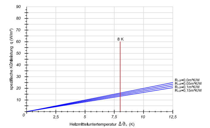
Verlegeabstand VA 350
