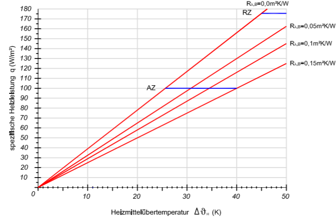
Verlegeabstand VA 150
