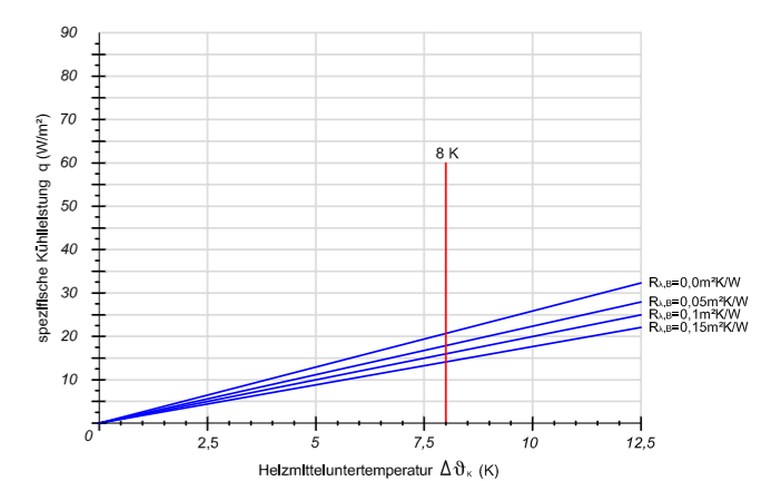
Verlegeabstand VA 350
