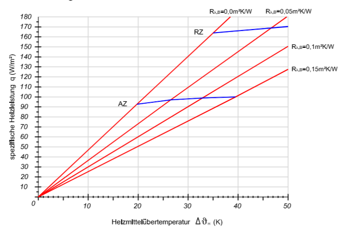
Verlegeabstand VA 200
