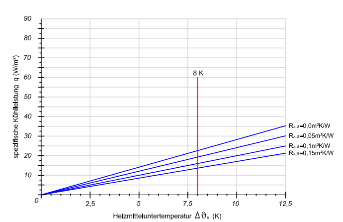
Verlegeabstand VA 300
