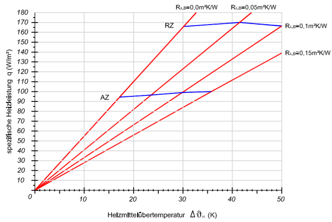
Verlegeabstand VA 150
