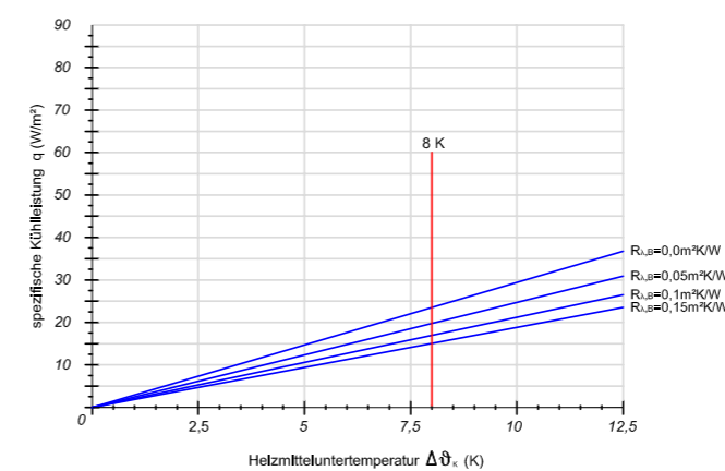
Verlegeabstand VA 300
