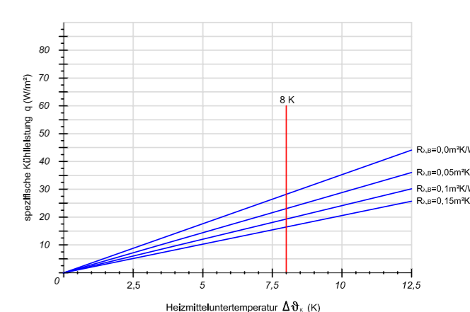
Verlegeabstand VA 200
