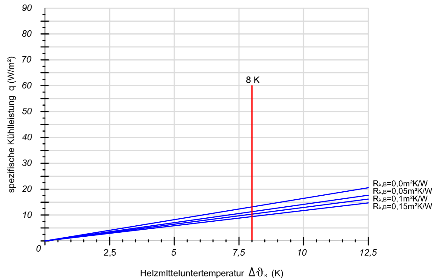
Verlegeabstand VA 125
