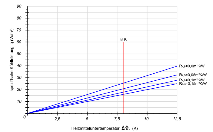
Verlegeabstand VA 250
