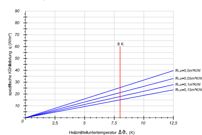
Verlegeabstand VA 250
