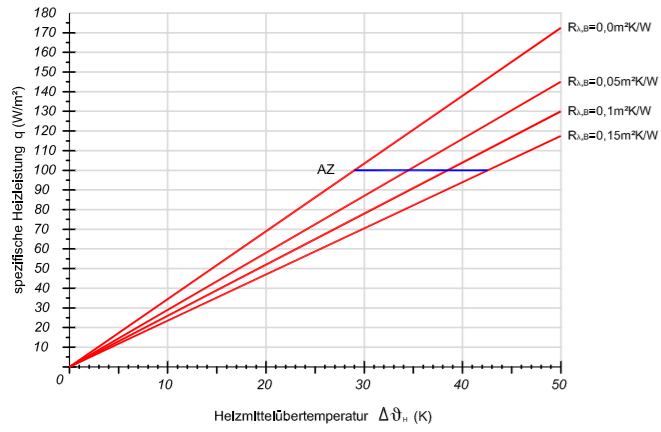
Verlegeabstand VA 200
