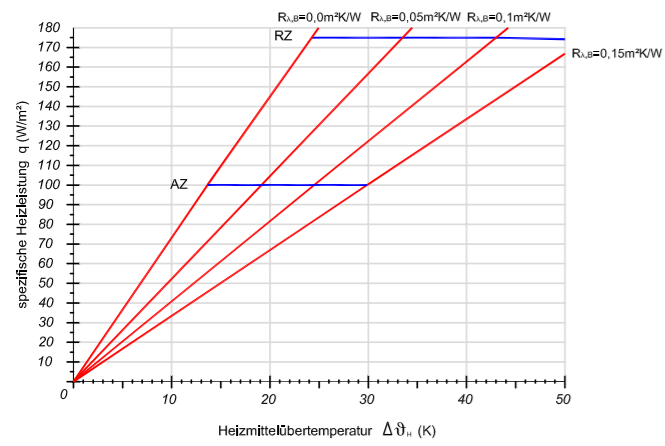
Verlegeabstand VA 50
