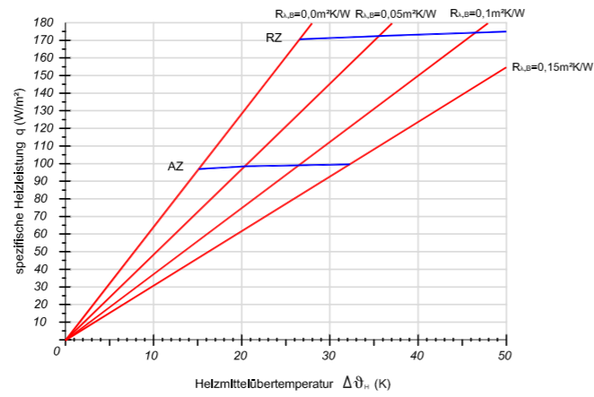
Verlegeabstand VA 100
