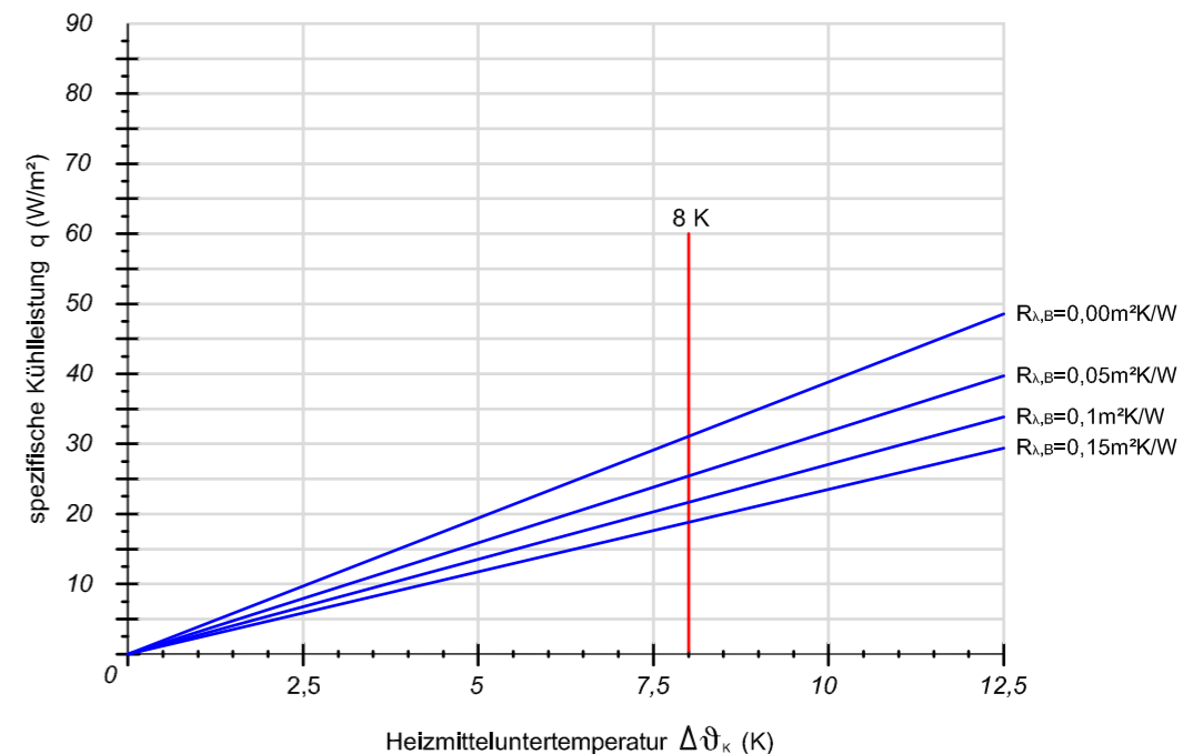
Verlegeabstand VA 125
