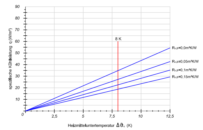
Verlegeabstand VA 100
