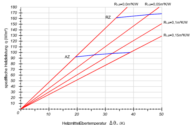
Verlegeabstand VA 200
