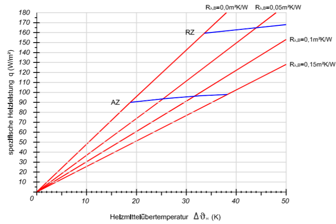
Verlegeabstand VA 200
