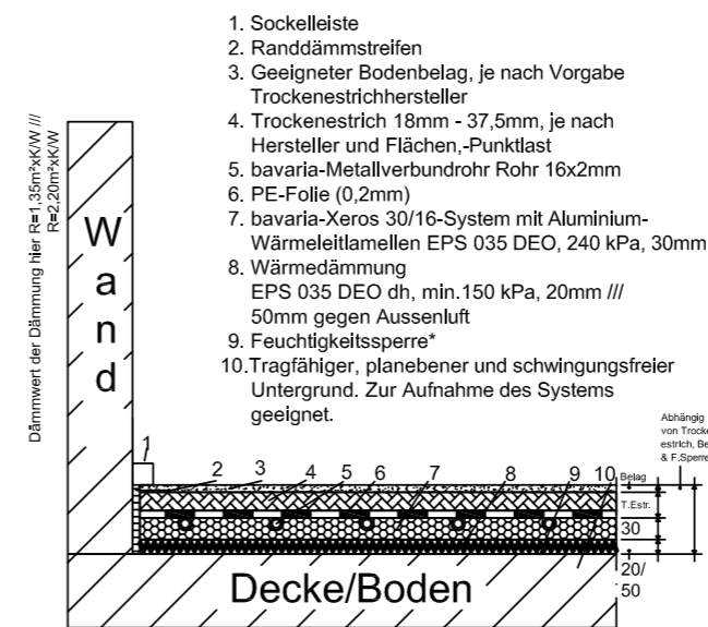
* Bauwerksabdichtung nach DIN 18195 nur gegen Erdreich / ** Höherer Dämmwert empfehlenswert / *** Bei Grundwasserspiegel < 5m höherer Dämmwert empfehlenswert Hinweis: Systemplatte keine Trittschallplatte. Gesamtaufbau z.B. mit Trockenestrich etc. erzeugt Trittschallverbesserung (Massivuntergrund). Holzunterkonstruktion immer situationbedngt.
