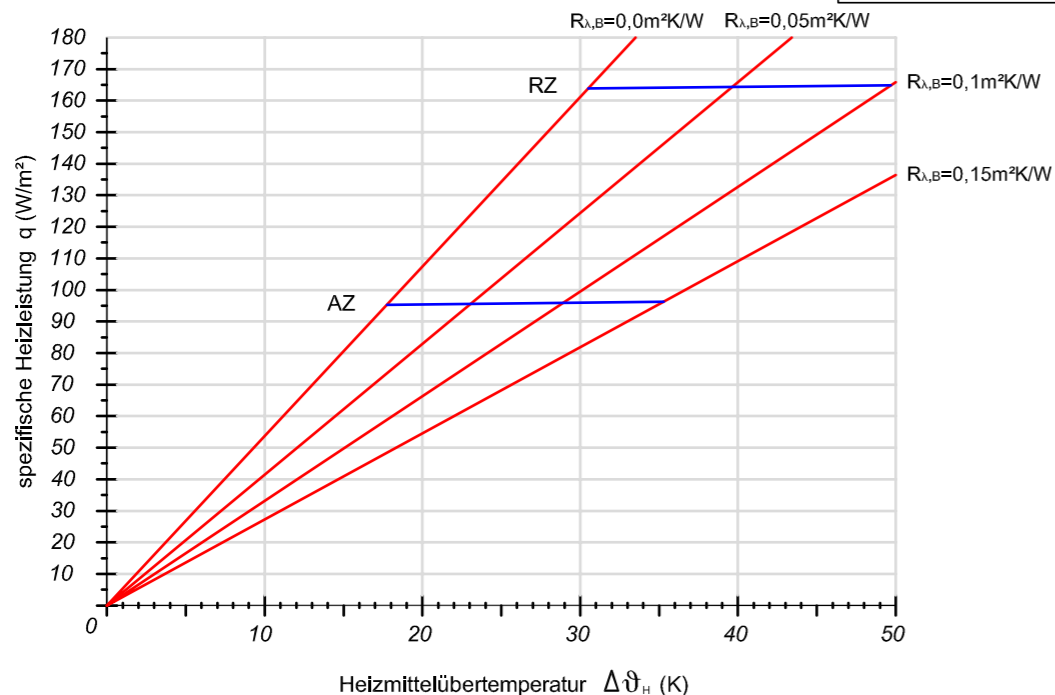
Verlegeabstand VA 125
