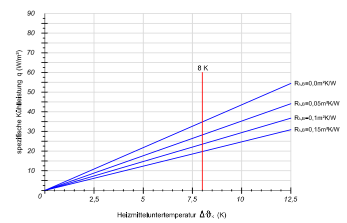
Verlegeabstand VA 100
