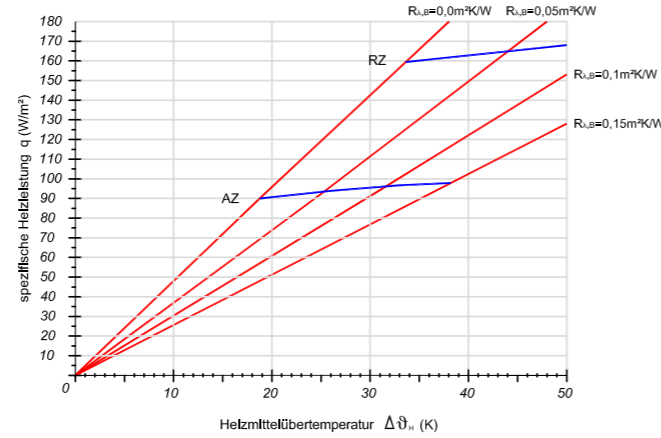
Verlegeabstand VA 200
