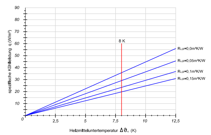
Verlegeabstand VA 100
