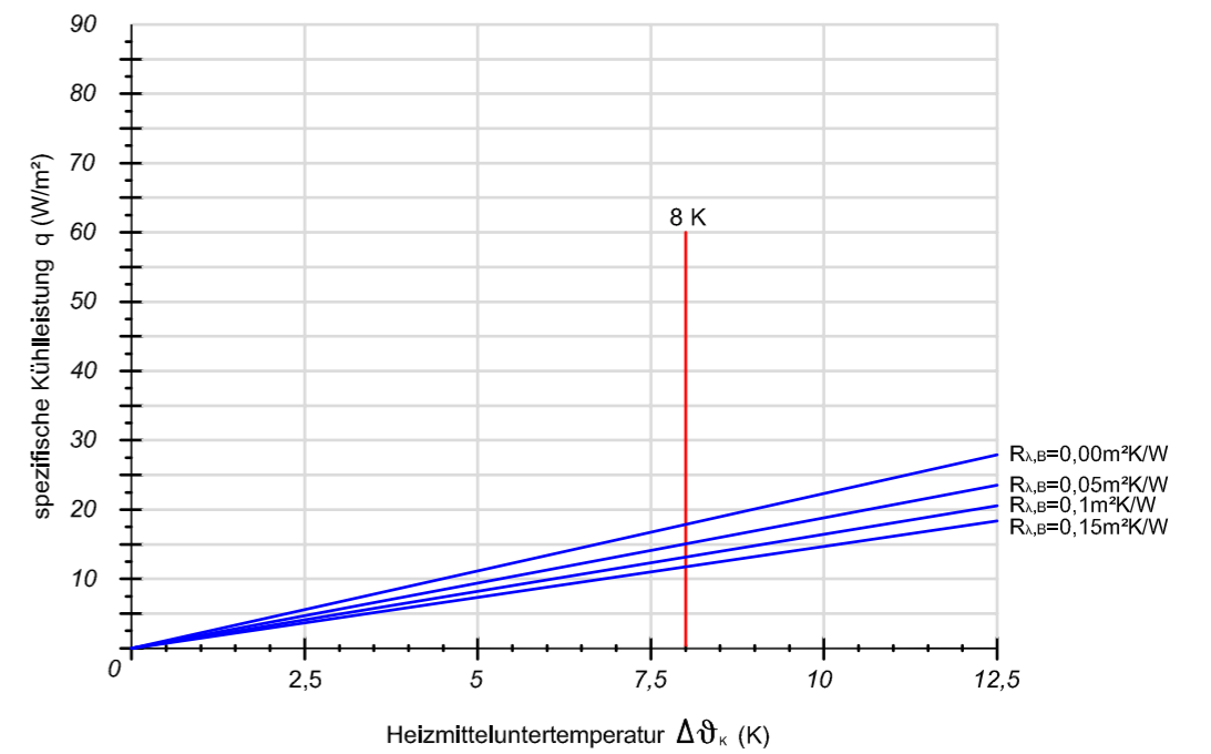
Verlegeabstand VA 250
