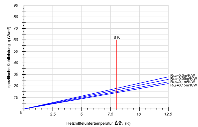
Verlegeabstand VA 300
