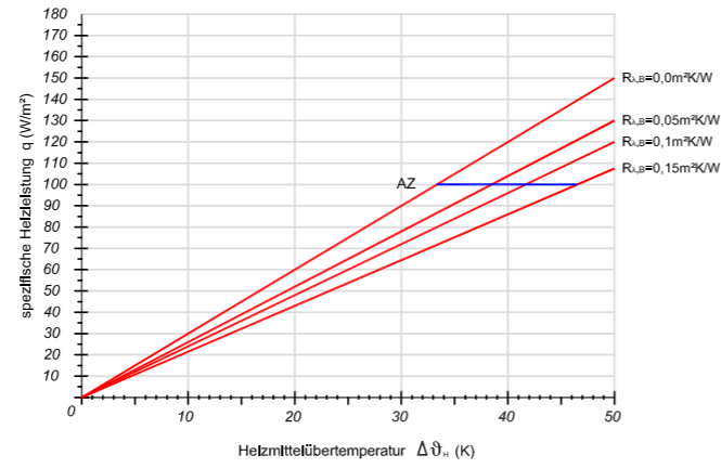
Verlegeabstand VA 250
