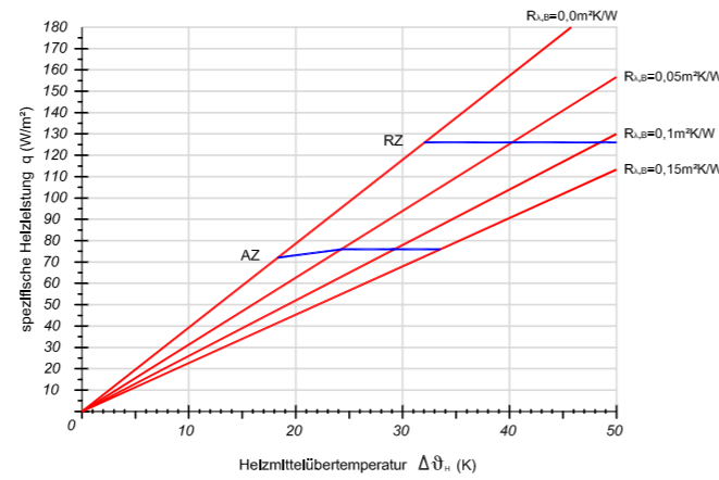
Verlegeabstand VA 250
