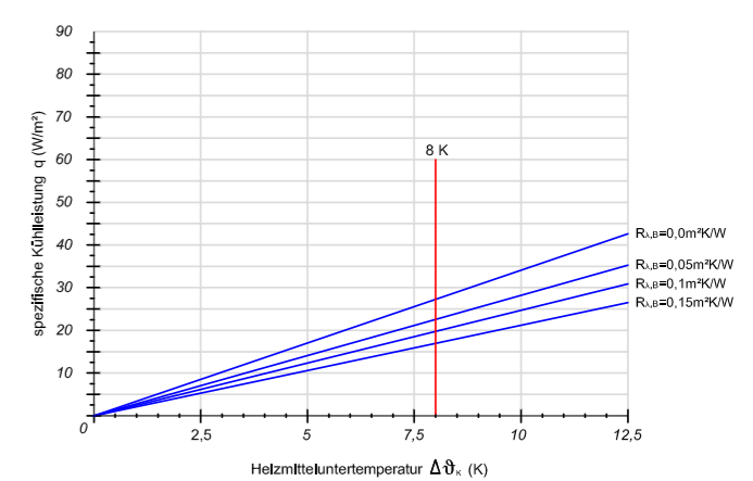
Verlegeabstand VA 250
