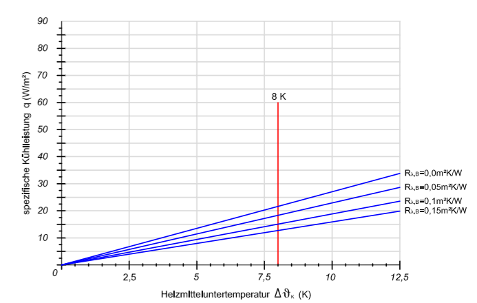
Verlegeabstand VA 300
