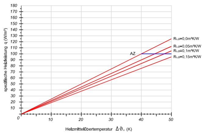
Verlegeabstand VA 300
